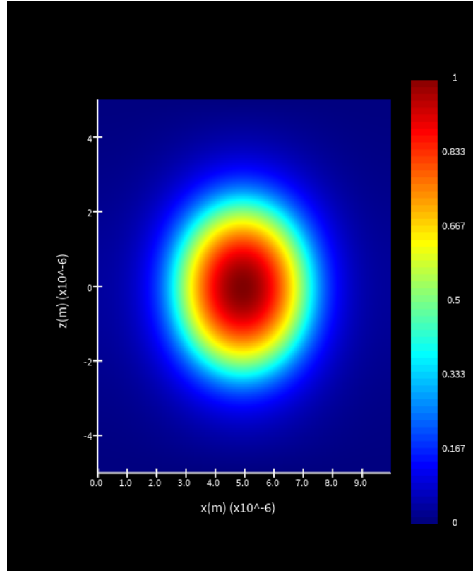
Fig. 5.11. Fibre Mode
