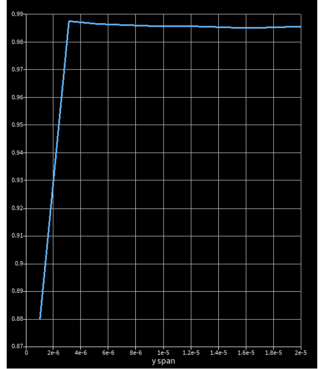
Fig. 6.12. Grating-Width 1
