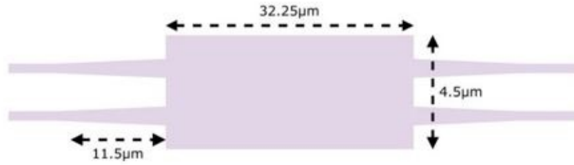
Fig. 4.10. MMI Geometry
