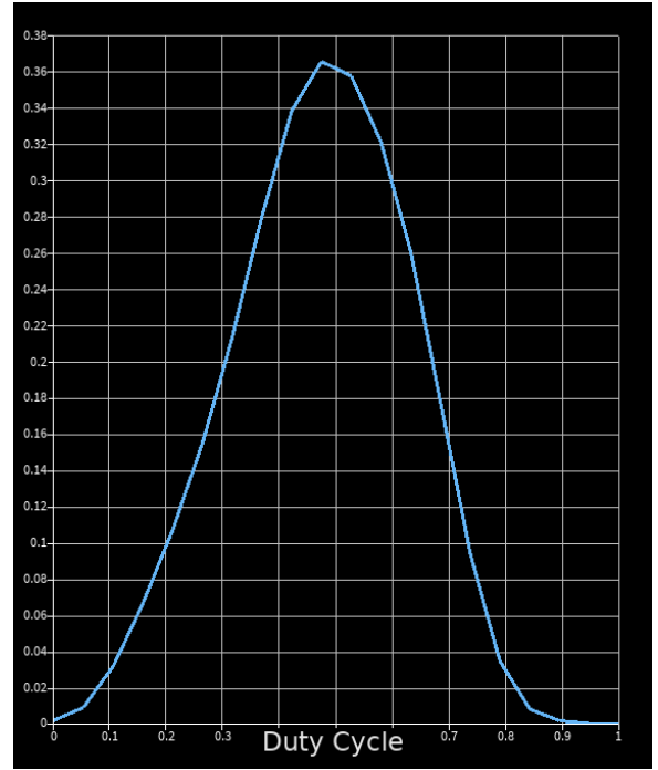
Fig. 5.6. Duty-cycle Sweep 1
