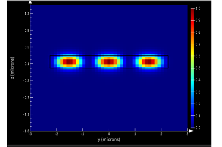
Fig. 4.7. 4.5 \mu\text{m} , TE Mode 3
